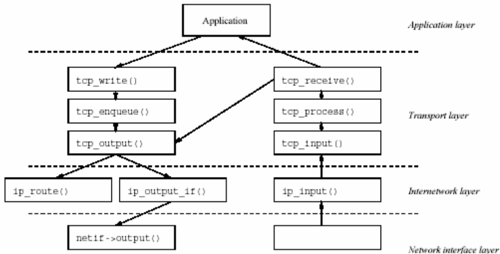
图 9 TCP 处理
