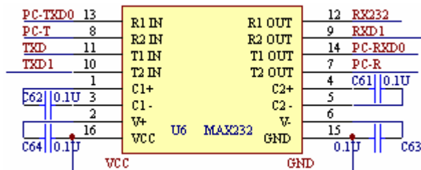
图 2.13.5 RS232 通讯电路
