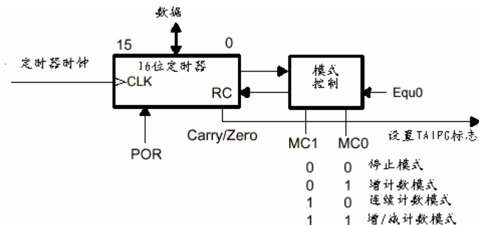
图 2.11.5 模式控制原理图
