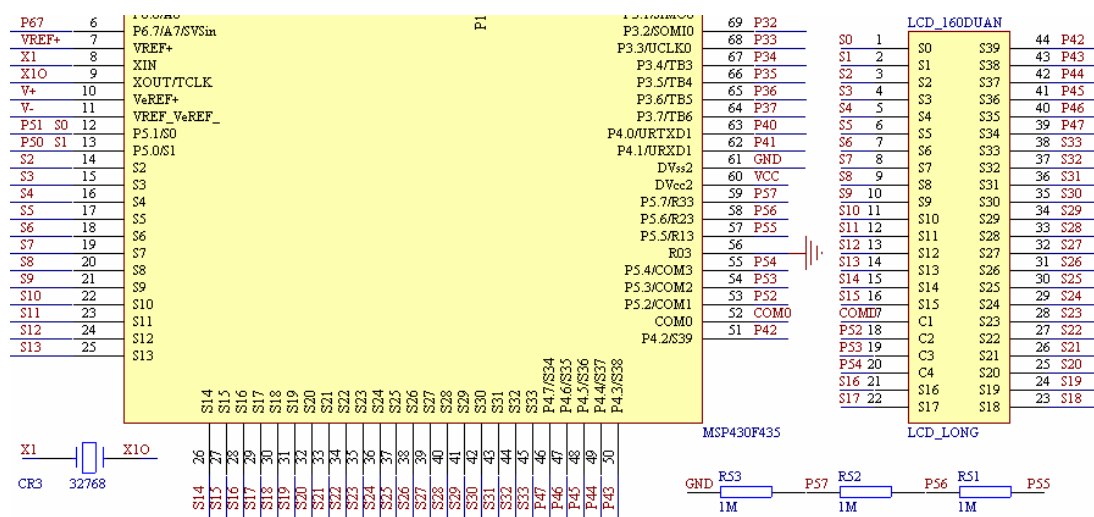
图 2.7.5 液晶显示电路
