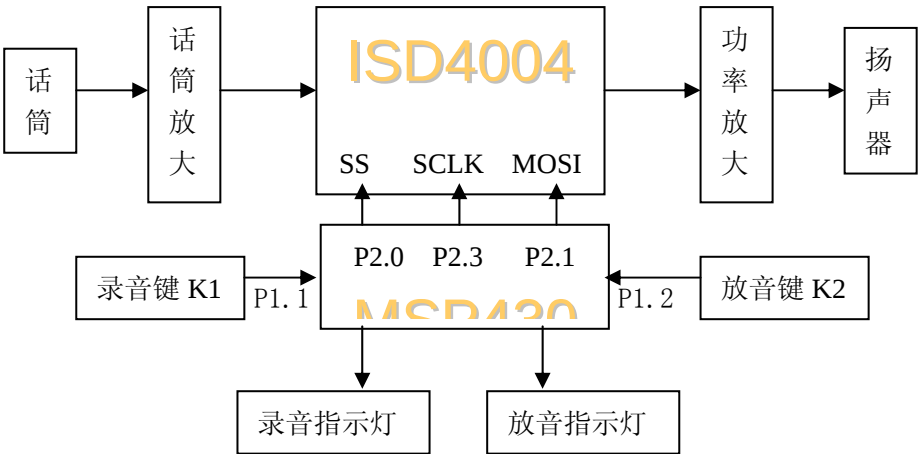
图 3. 10. 3 固体录音机电路框图
