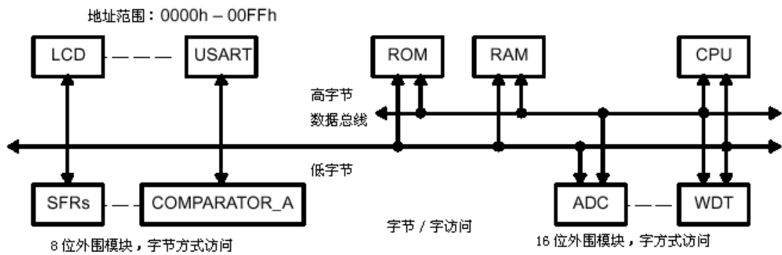
图 2.3 各种模块与总线的连接
