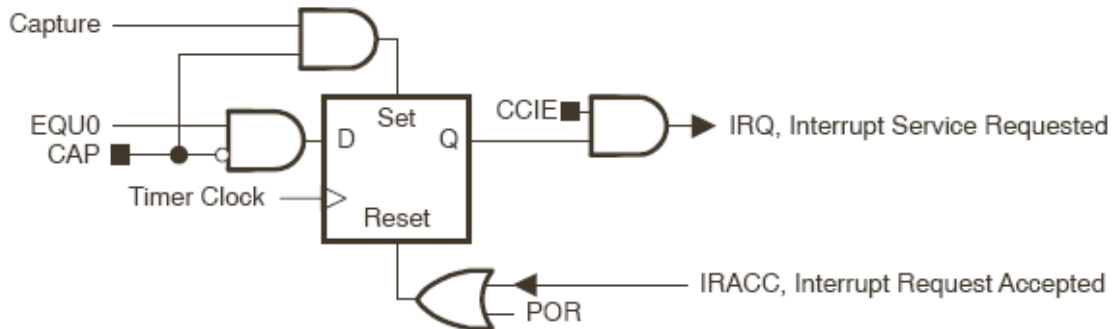
图 8-15 捕获比较 TACCR0 中断标志
