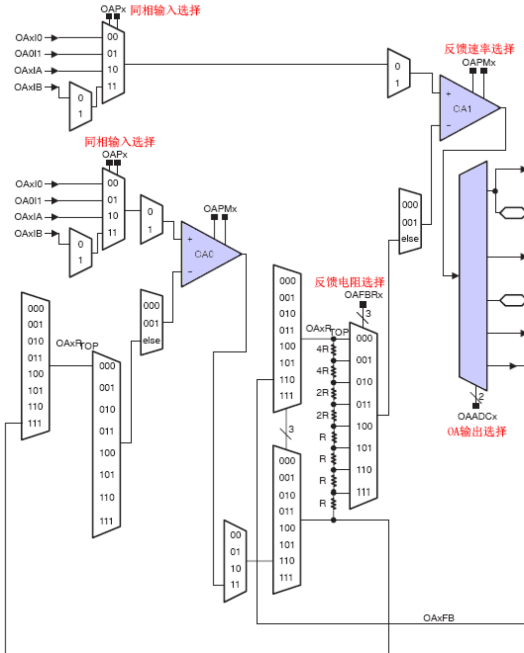
图 14-3 两运放差分放大器 OAx 相互连接
