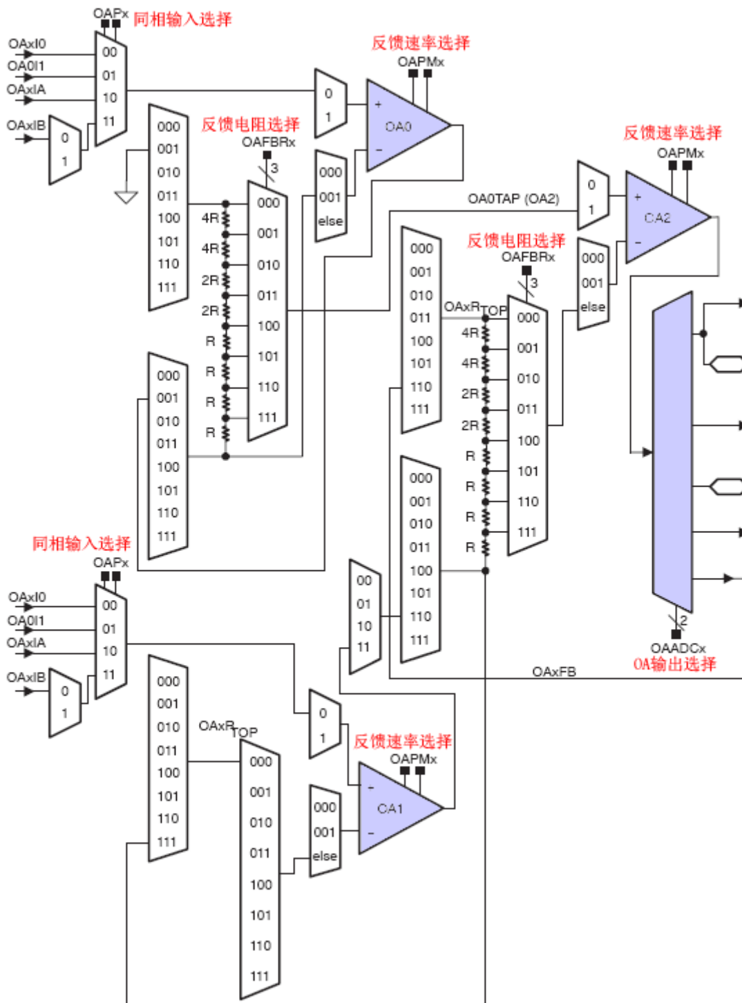
图 14-5 三运放差分放大器 OAx 相互连接
