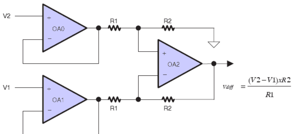
图 14-4 三运放差分放大器
