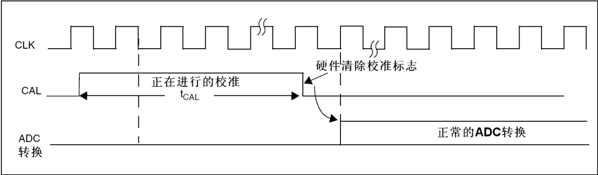
图28 校准时序图
