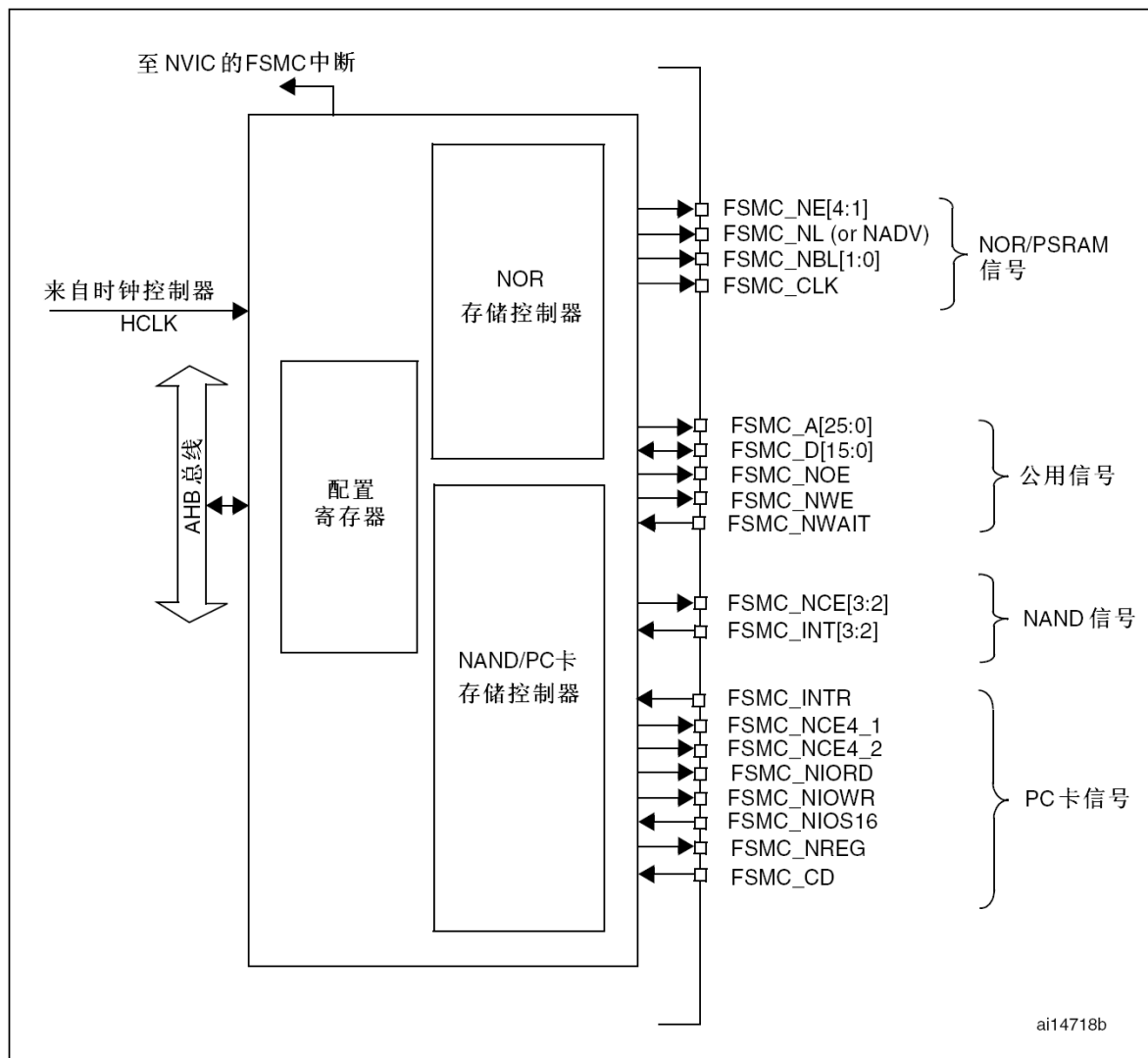
图160 FSMC框图
